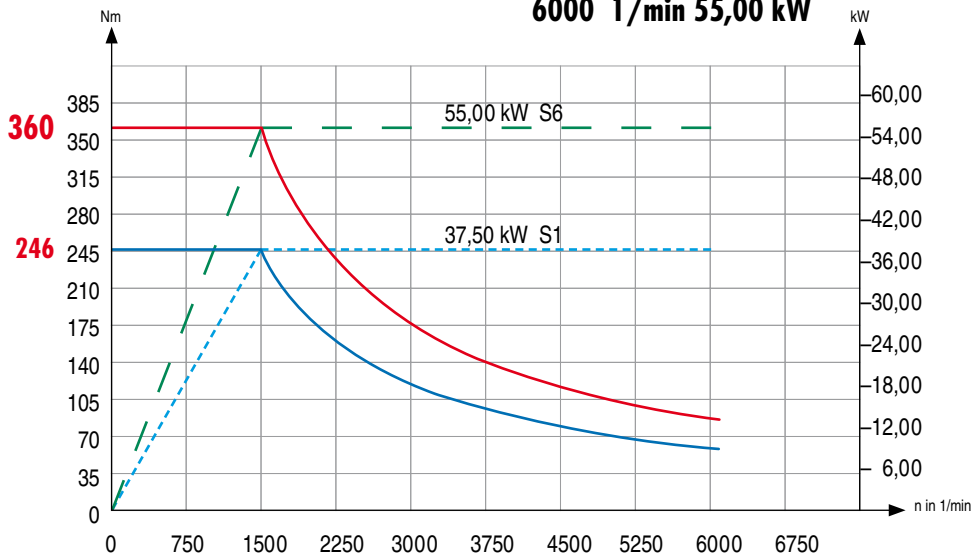
6000 1/min 55,00 kW
