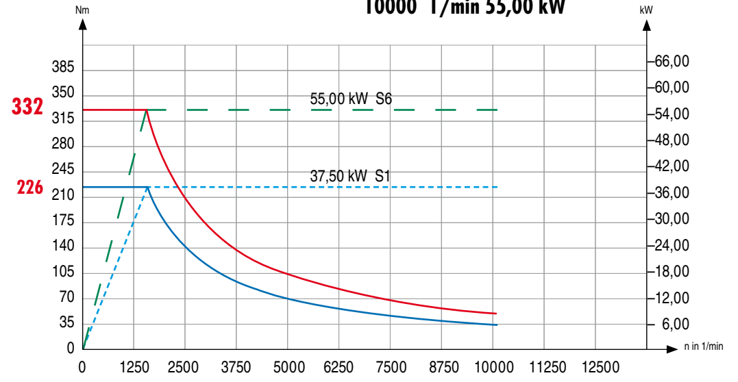
10000 1/min 55,00 kW
