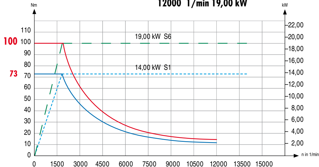
12000 1/min 19,00 kW
