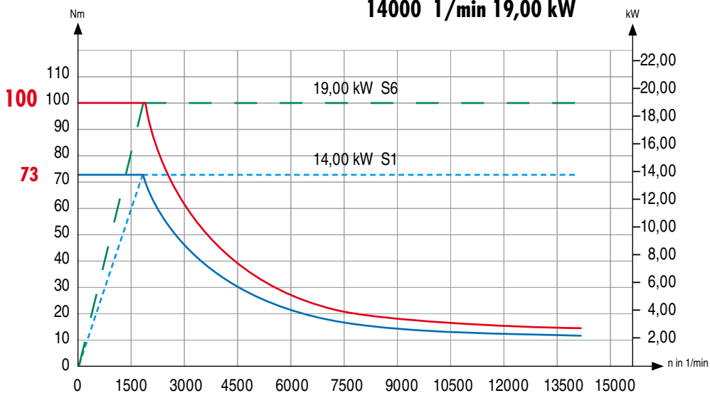
14000 1/min 19,00 kW
