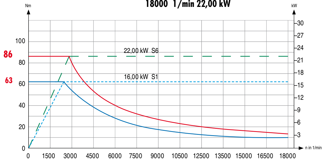
18000 1/min 22,00 kW
