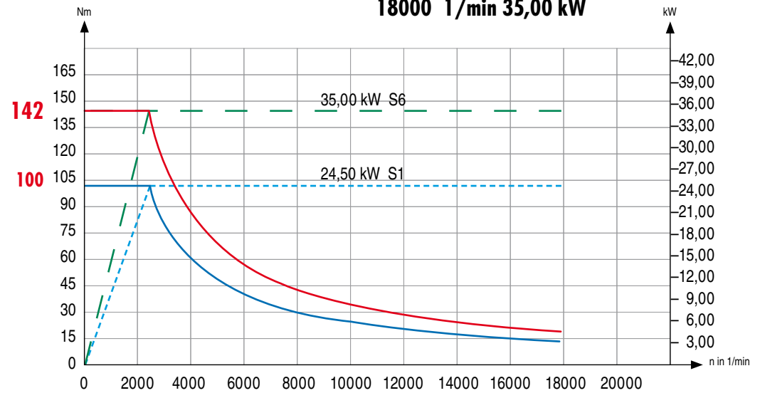
18000 1/min 35,00 kW
