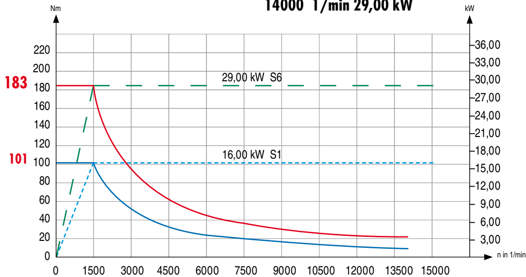
14000 1/min 29,00 kW
