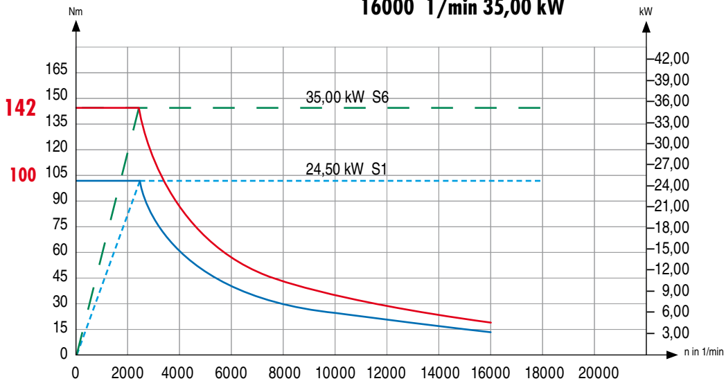
16000 1/min 35,00 kW
