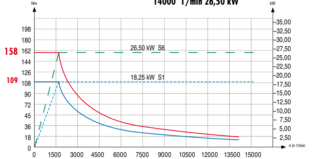
14000 1/min 26,50 kW
