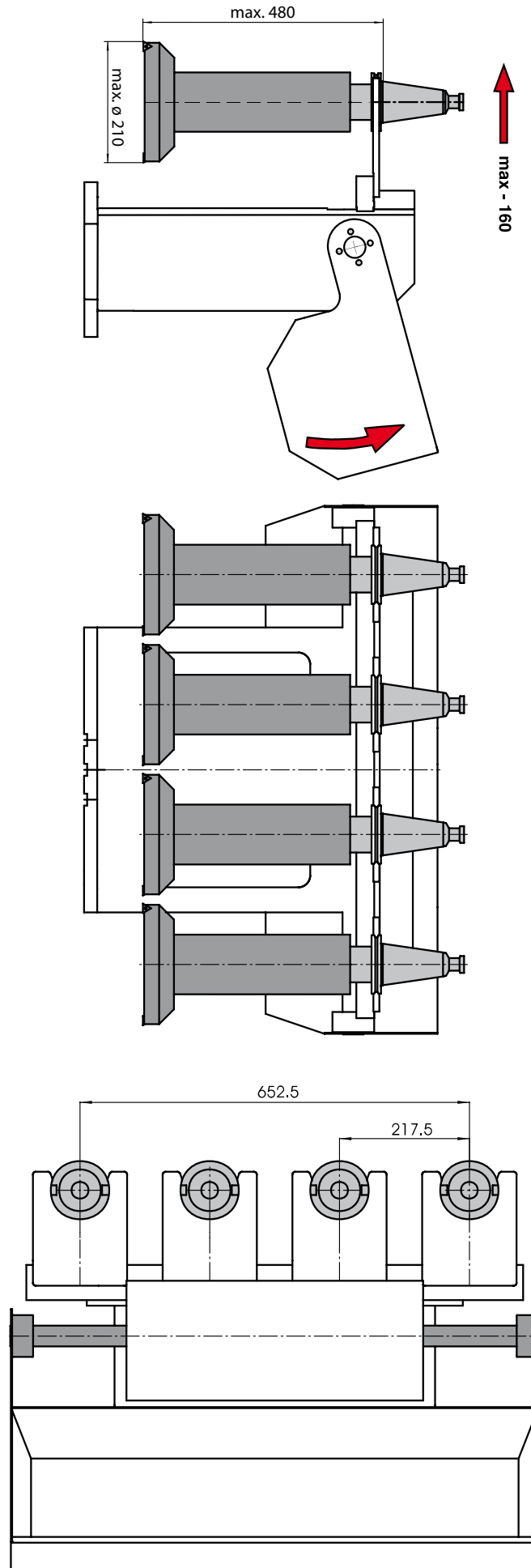
BOVENAANZICHT
