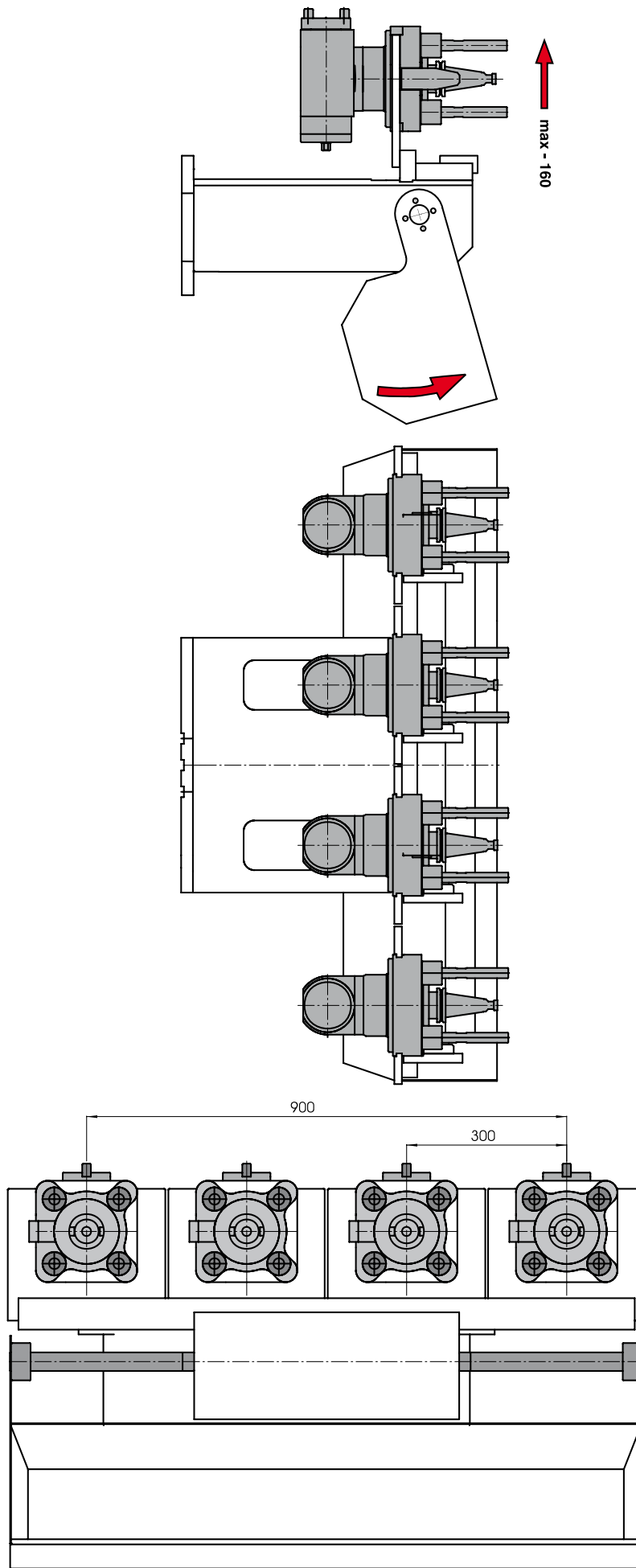
BOVENAANZICHT
