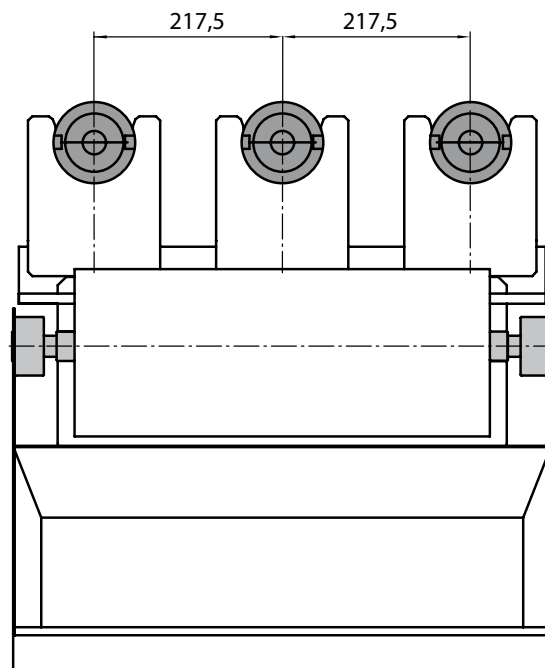
BOVENAANZICHT
