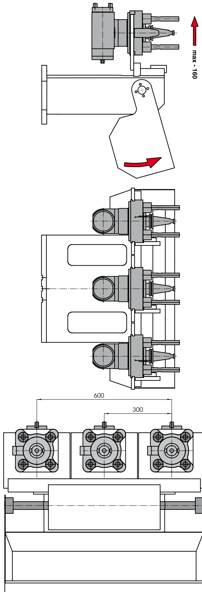
BOVENAANZICHT
