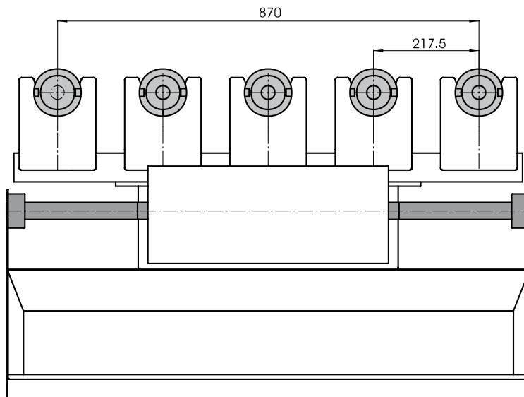
BOVENAANZICHT
