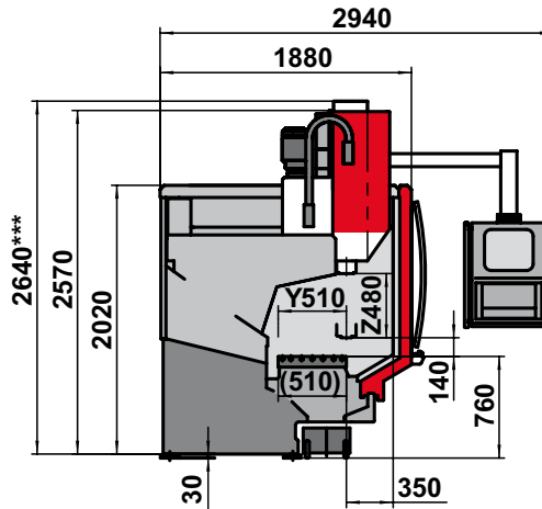
Z-Schlitten-Kontur bei Celox Z-Schlitten-Kontur bei ISO 40
